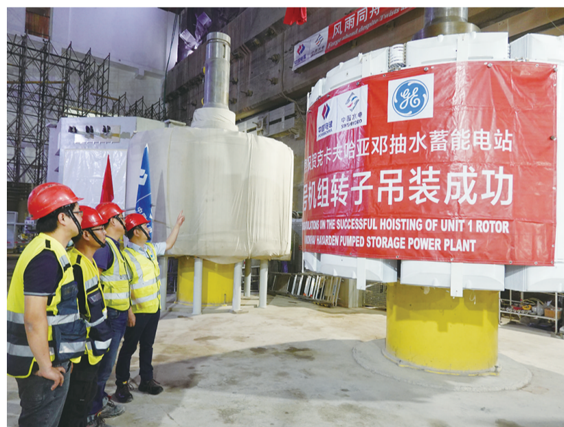
5月25日,在以色列东北部贝特谢安市的抽水蓄能电站建设现场,中国电建工作人员进行1号机转子吊装作业。该电站位于以色列东北部贝特谢安市,毗邻约旦河谷,机组位于海平面以下275米,总装机容量预计达344兆瓦,建成后将成为全球海拔最低、以色列规模最大的抽水蓄能电站,预计2023年年初完工投产。
